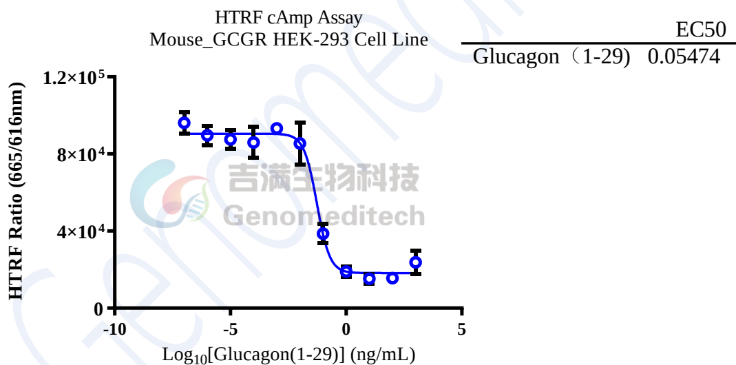
Fig 2. 将 Mouse_GCGR HEK-293 细胞以 7500 cells/孔 的密度接种于 白色 384 孔微孔板 (5 \mu L/孔) 中。随后添加梯度稀释的人 Glucagon(1-29)溶液, 并在室温下孵育 30 min。然后使用 HTRF cAMP Gs Dynamic Detection Kit (revvity/62AM4PEB) 按照厂商说明书进行检测, 使用 Molecular Devices i3x 多功能读板仪, 以 340 nm 激发光、在 616 nm 和 665 nm 波长下测定发射信号。信号值以 665 nm/616 nm * 100000 (HTRF Ratio) 表示, 并用于计算 EC50 值。
